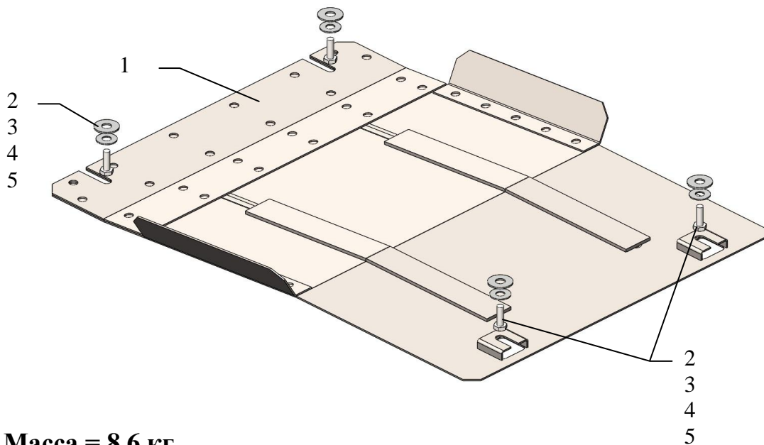
Схема сборки защиты КПП.
